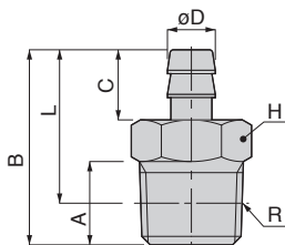
管用テーパネジの場合
